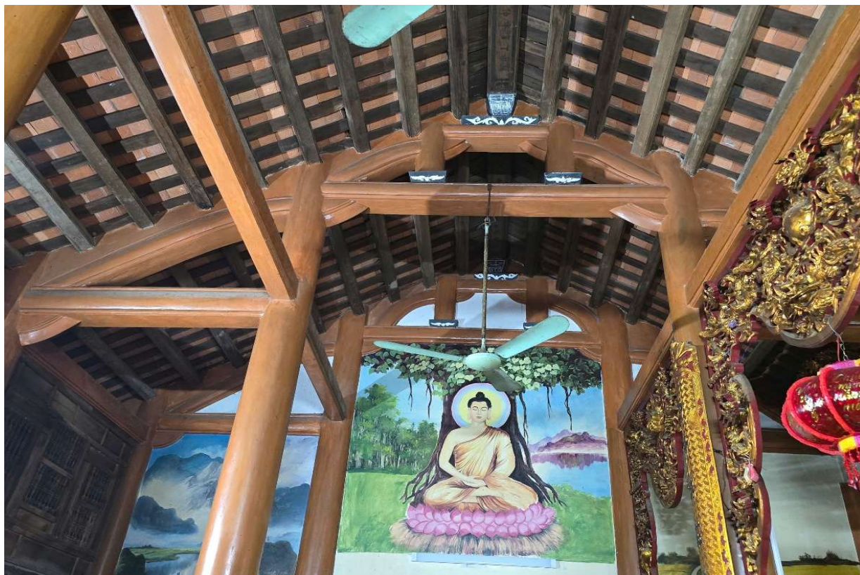
BỘ VÌ TRỤC 3 NHÀ MẪU (BÊ TÔNG SƠN GIẢ GỖ)
